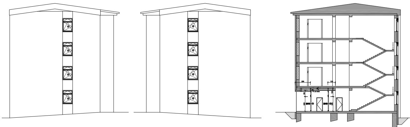
VÝCHODNÝ POHĽAD
