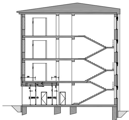
REZ A-A
